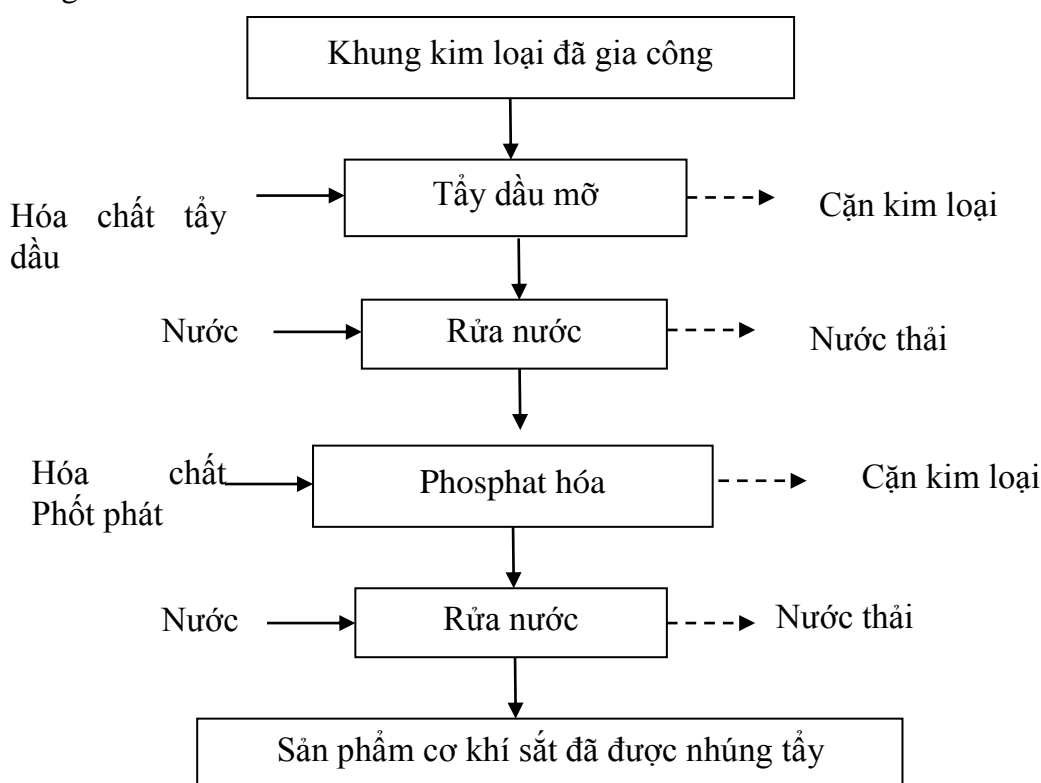
Hình I.5. Quy trình nhúng tẩy kim loại
