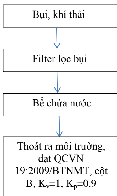
Hình IV.1. Sơ đồ xử lý bụi sơn tĩnh điện
