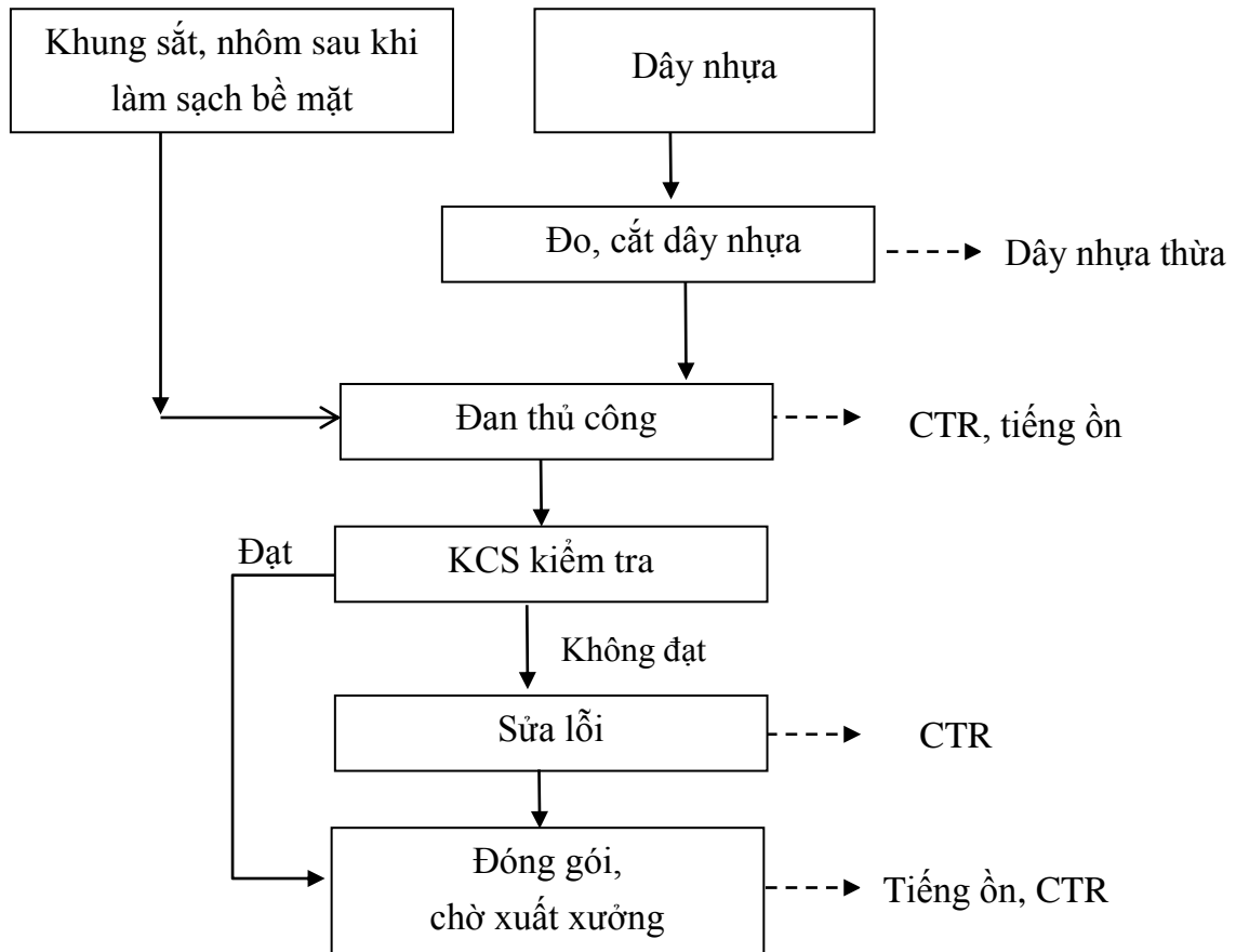
Hình I.7. Sơ đồ quy trình sản xuất bàn ghế đan nhựa giả mây
