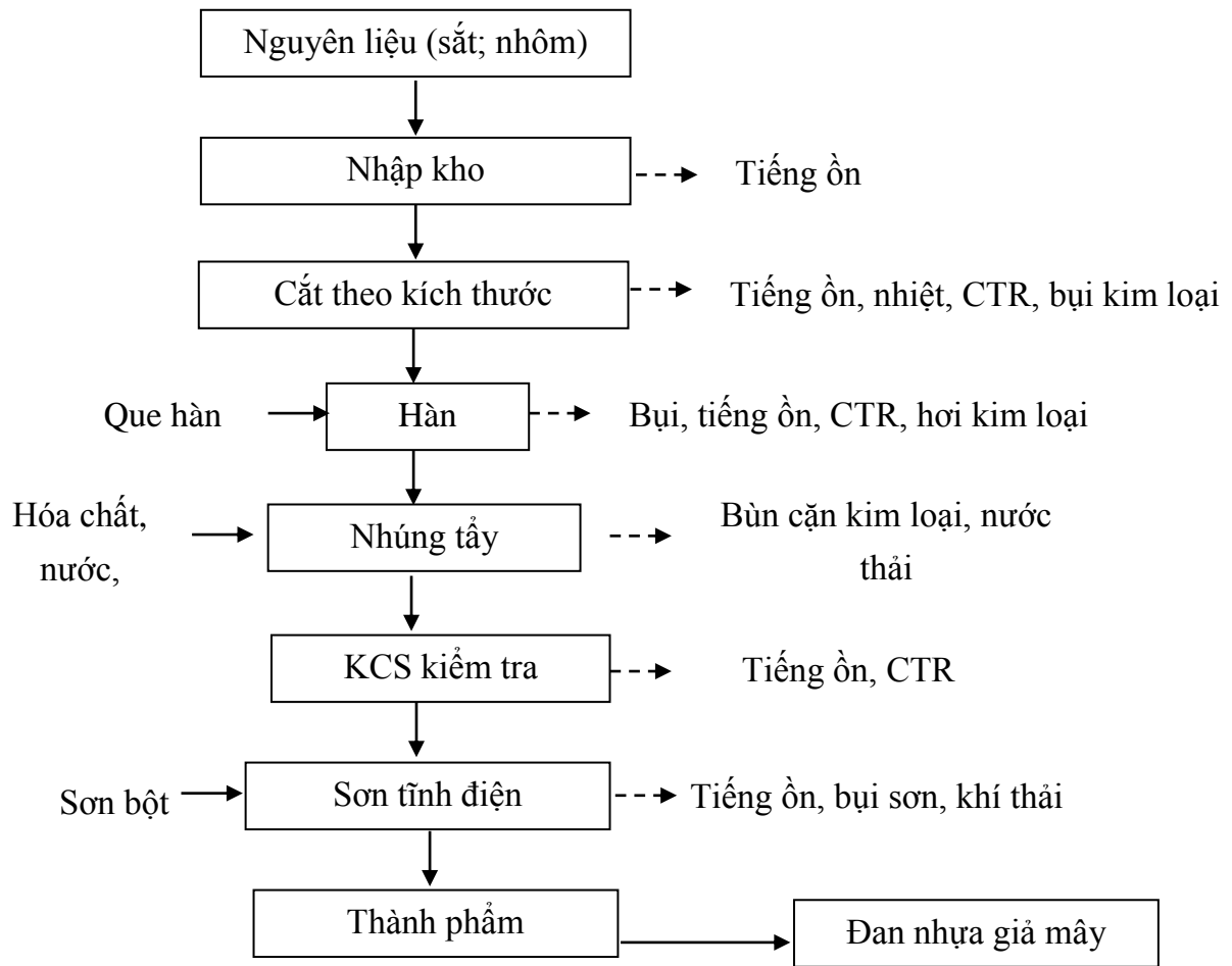
Hình I.4. Sơ đồ quy trình gia công cơ khí
