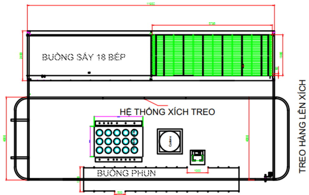
Hình IV.3. Sơ đồ bố trí hệ thống phun sơn tĩnh điện
