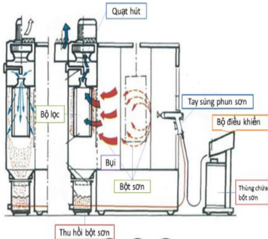
Hình IV.2. Sơ đồ hệ thống Filter lọc bụi được lắp đặt đồng bộ trong buồng sơn tĩnh điện
