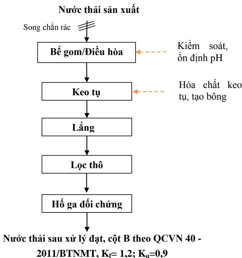
Hình IV.5. Quy trình công nghệ xử lý nước thải sản xuất
