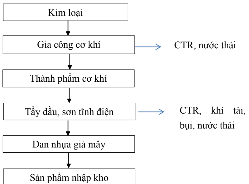
Hình I.3. Sơ đồ quy trình sản xuất sản phẩm nội thất từ kim loại đan nhựa giả mây
