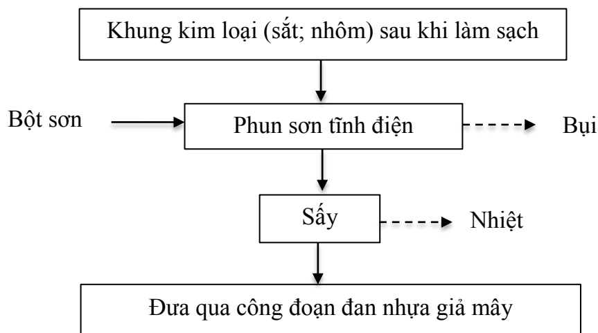
Hình I.6. Sơ đồ quy trình sơn tĩnh điện
