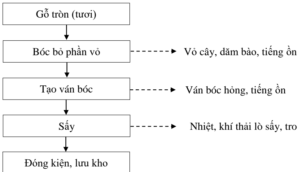
Hình 1.2. Quy trình công nghệ sản xuất ván bóc tại dự án
