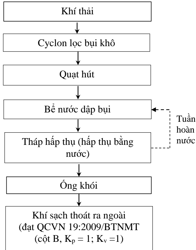
Hình 4.7. Quy trình công nghệ xử lý khí thải lò hơi sấy gỗ thanh
