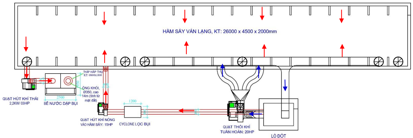
Hình 4.6. Sơ đồ mặt bằng bố trí hệ thống xử lý khí thải lò sấy ván bóc
