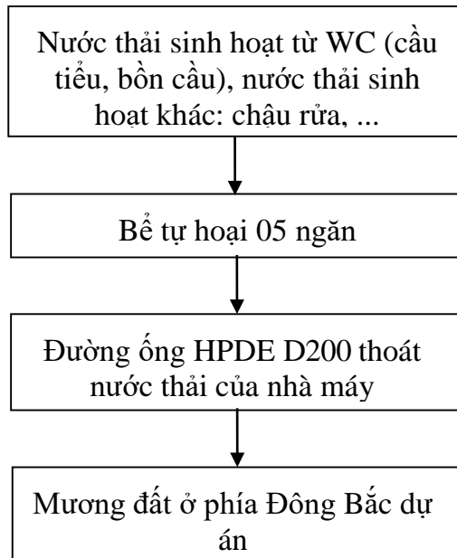
Hình 4.1. Sơ đồ thu gom, thoát nước thải sinh hoạt của dự án
