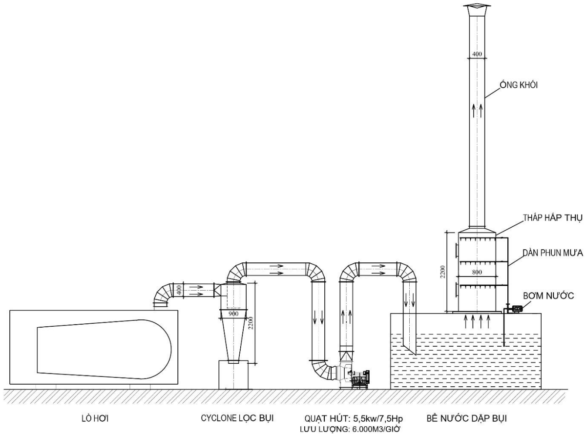
Hình 4.8. Sơ đồ bố trí hệ thống xử lý khí thải lò hơi
