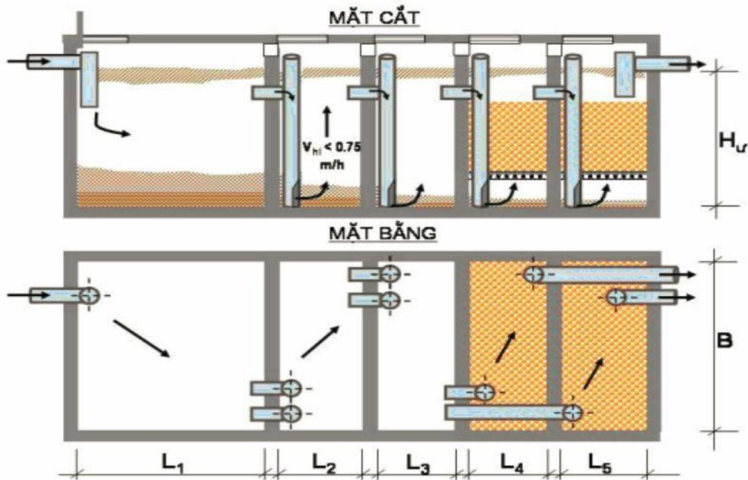
Hình 4.3. Sơ đồ mô hình bể tự hoại 05 ngăn
