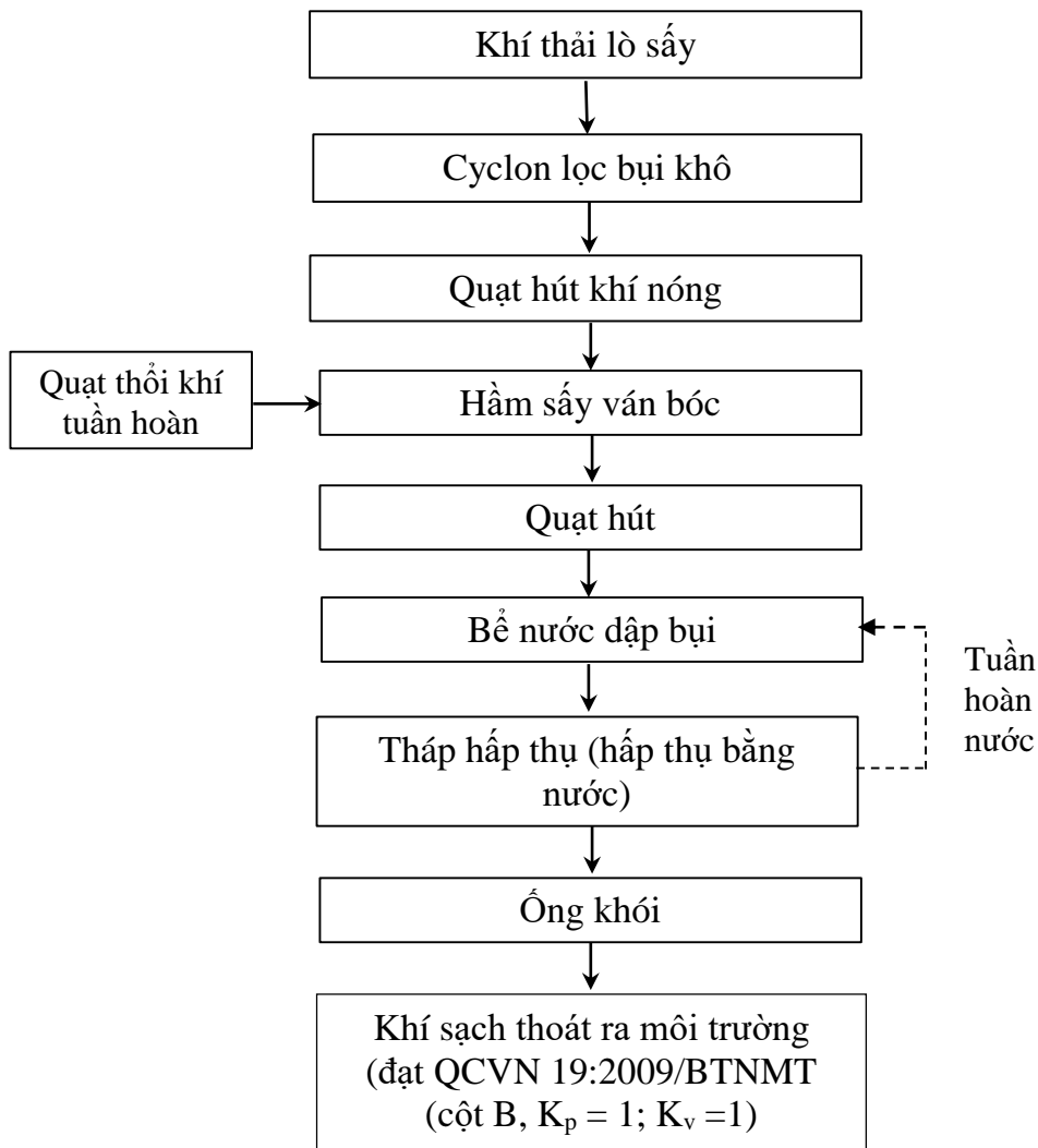
Hình 4.5. Quy trình công nghệ xử lý khí thải lò sấy ván bóc
